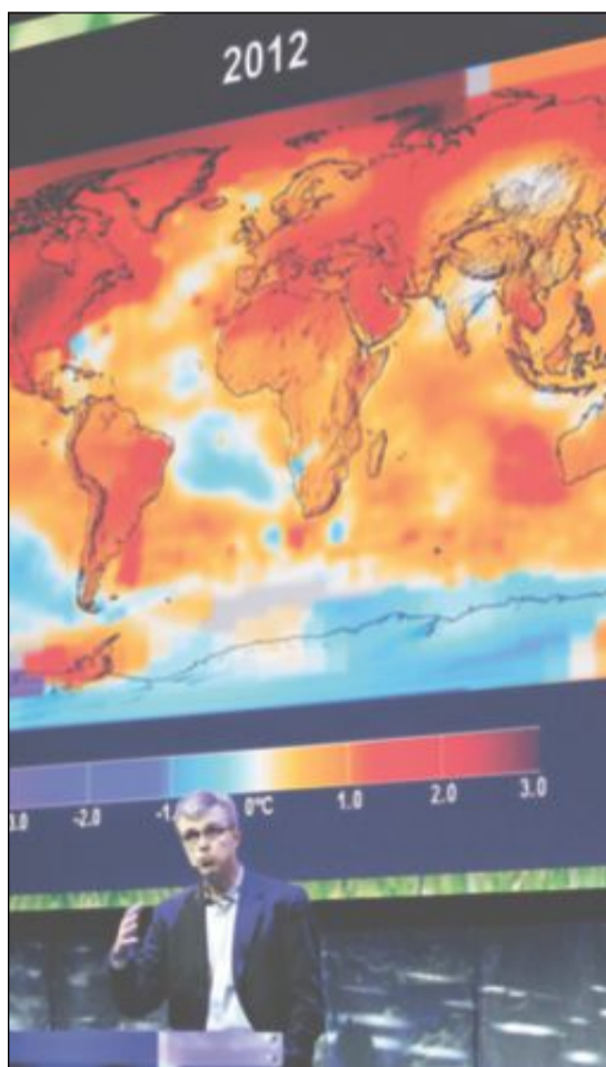
VISER JORDENS TEMPERATUR: Helge Drange, forsker ved Bjerkesenteret og professor ved Geofysisk institutt ved Universitetet i Bergen, viste i sitt foredrag et skremmende bilde av hva som har skjedd temperaturemessig siden begynnelsen av 1900-tallet og hvor fort utviklingen går mot en enda varmere verden.
